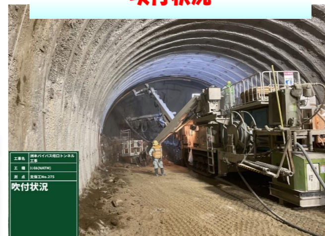
L=278.9m地点
